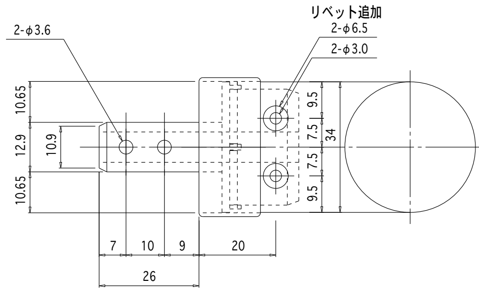
Z矢视图 (リベット詳細図)
